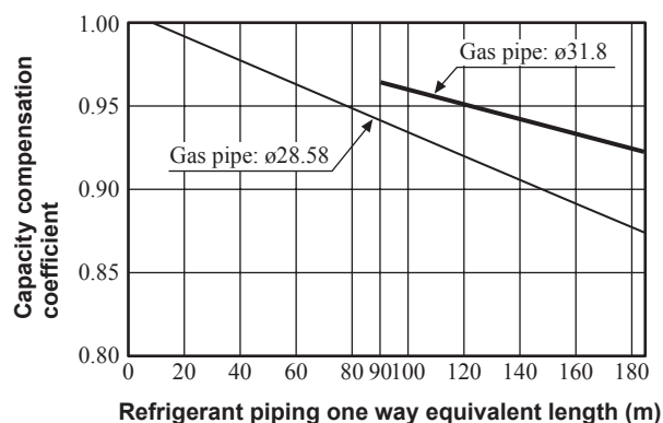
Model FDC(S)615KXZE1 (FDC(S)280KXZE1 + FDC(S)335KXZE1)
